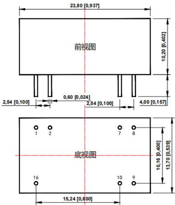
外观尺寸图
