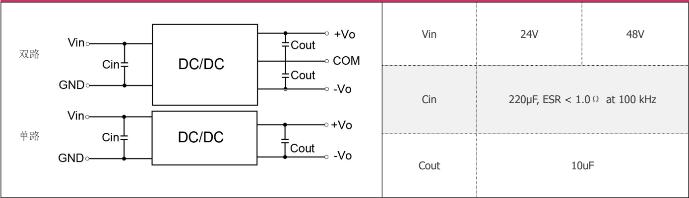
应用电路（图 2）
