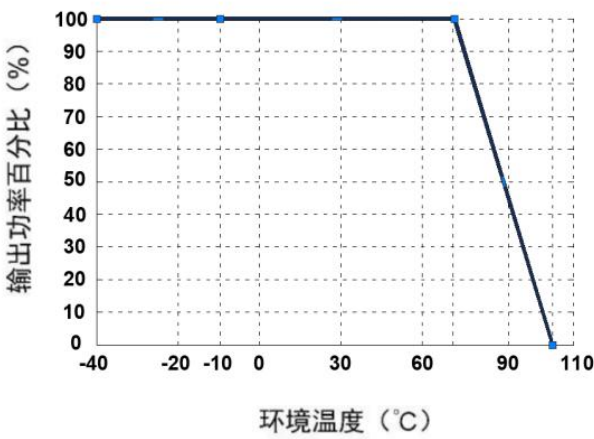
温度降额曲线图（图 1）
