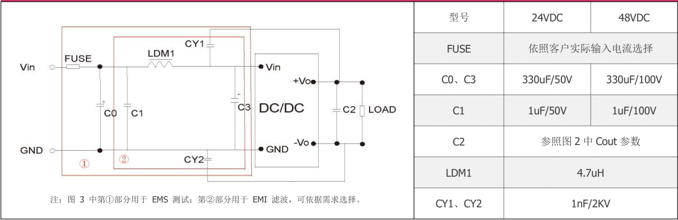
应用电路（图 3）
