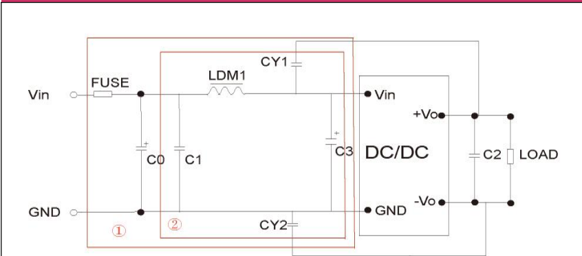
应用电路（图 3）
