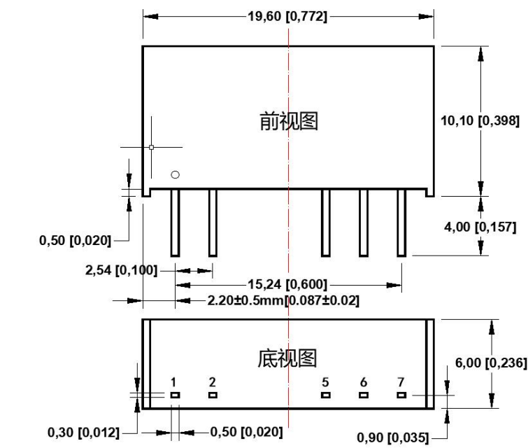
外观尺寸图
