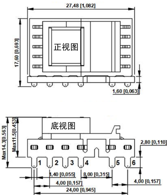
AWS05-23Sxx-F 外观尺寸图
