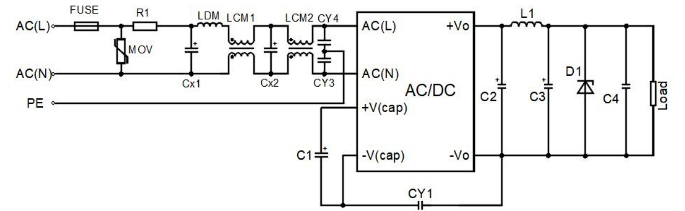
EMC 推荐电路
