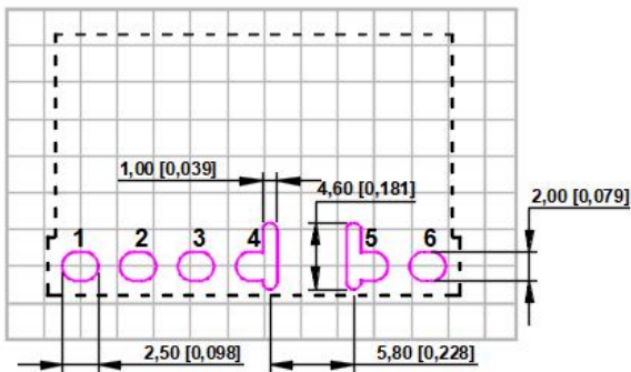
PCB 印刷版图
